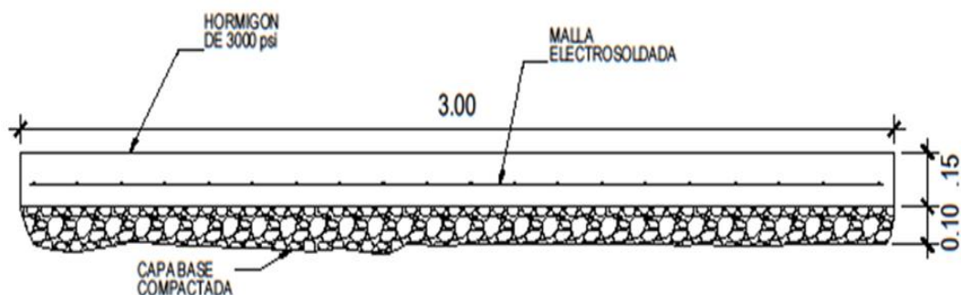
DETALLE TÍPICO DE VEREDA CALLE ESC: 1:10
