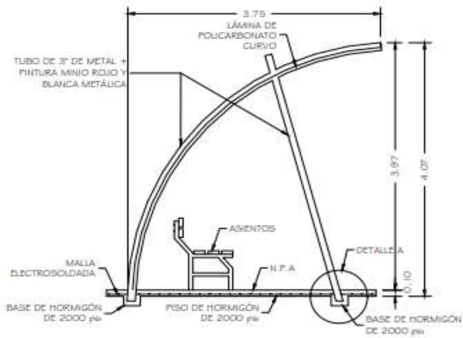
SECCIÓN I ESC.: 1:100
