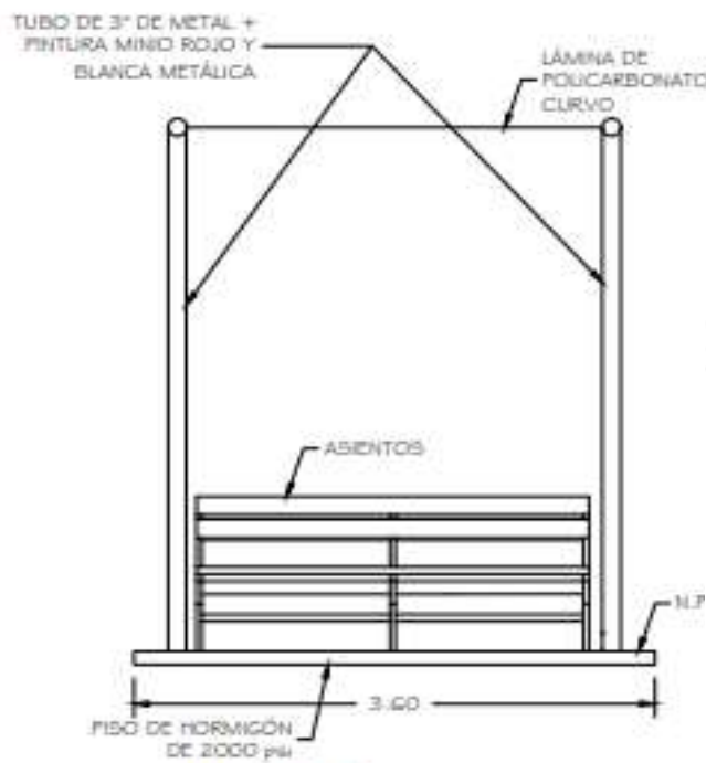
ELEVACIÓN FRONTAL ESC.: 1:100
