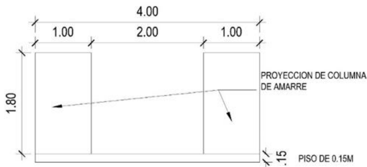
ELEVACION FRONTAL
