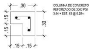
DETALLE CL
