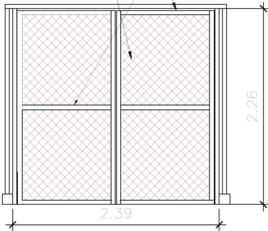
DETALLE DE PUERTA DE ACCESO
