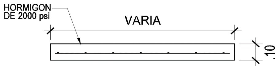
DETALLE TIPICO DE VEREDA ESC.: 1/10
