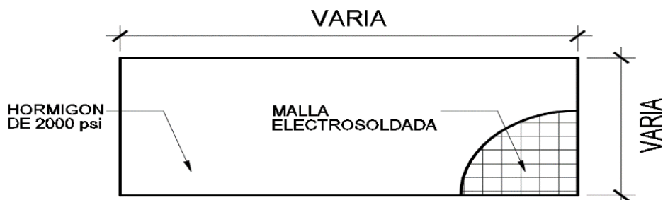
DETALLE TIPICO DE VEREDA ESC.: 1/10
